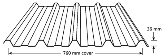
(ROOF SPAN TABLE - 0.42MM)
