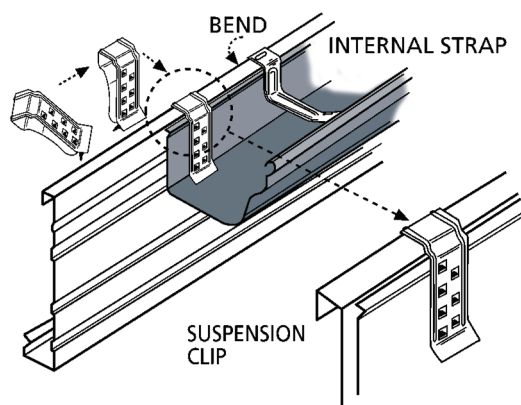
115 OG - STEEL FASCIA
