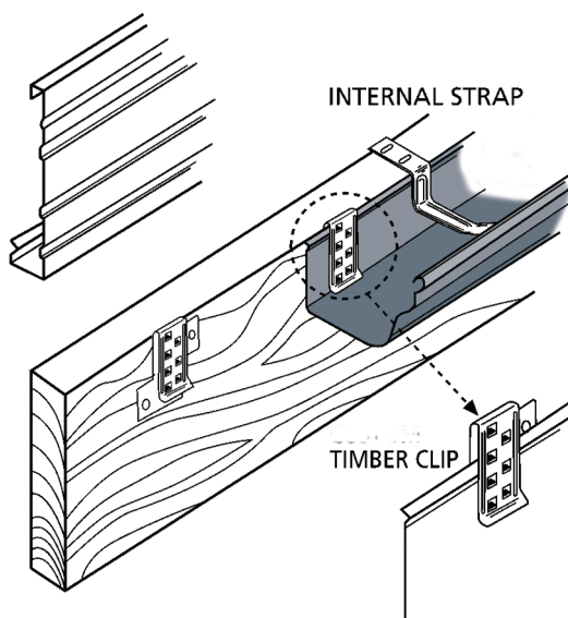
115 OG TIMBER OR STEEL FASCIA
